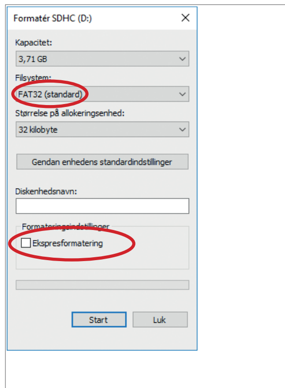
Trin 2
