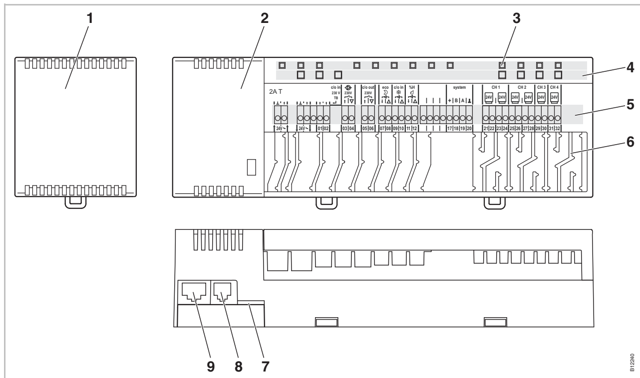
Fig. 2: Utformning av kontrollenheten, figuren visar 4-kanalversionen.
