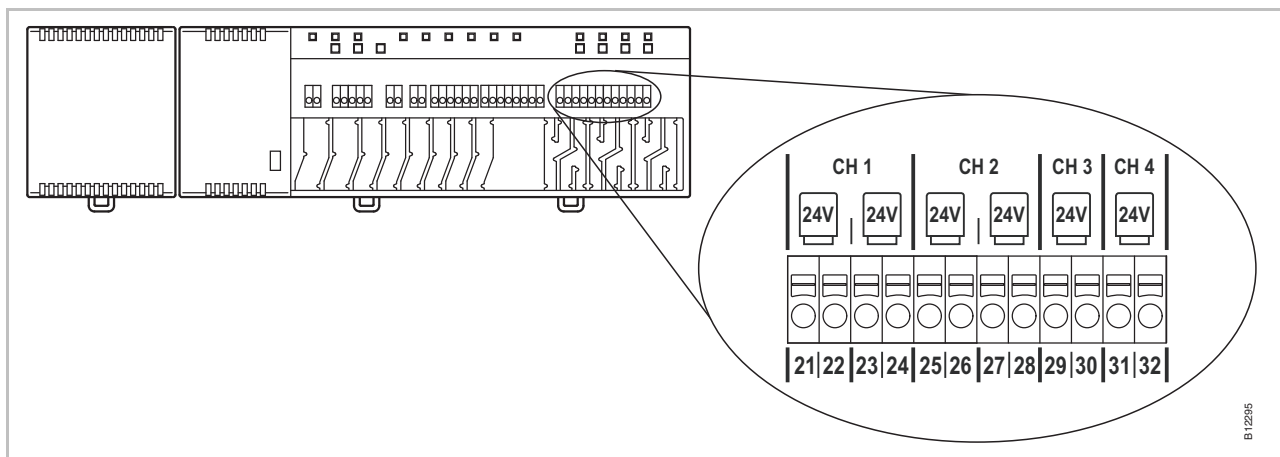
Fig. 25: Anslutning av reglermotorer
