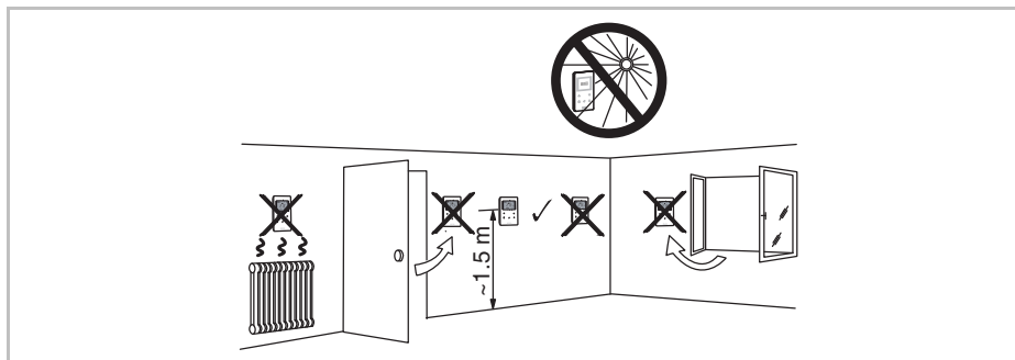
Fig. 9: Monteringsinstruktioner
