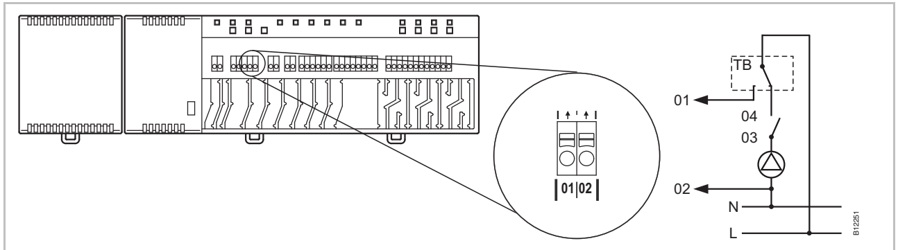
Fig. 28: TB-ingång för temperaturövervakning
