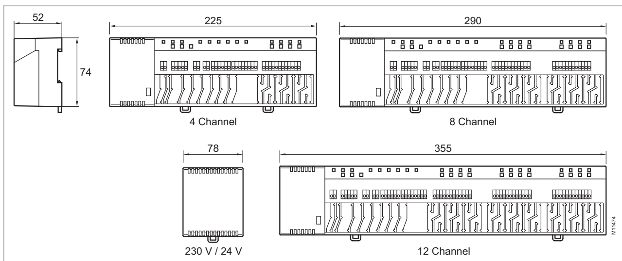
Fig. 41: Mått för kontrollenhet med transformator (alla mått i mm)
