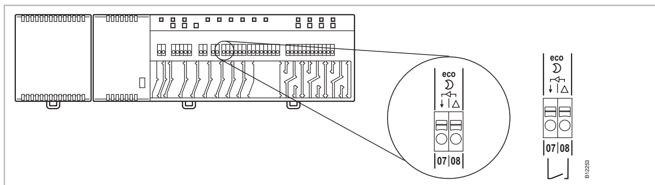
Fig. 30: Eko-ingång, kontaktdetektion
