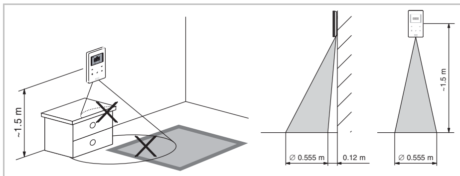
Fig. 10: Verkningsgrad IR-sensor
