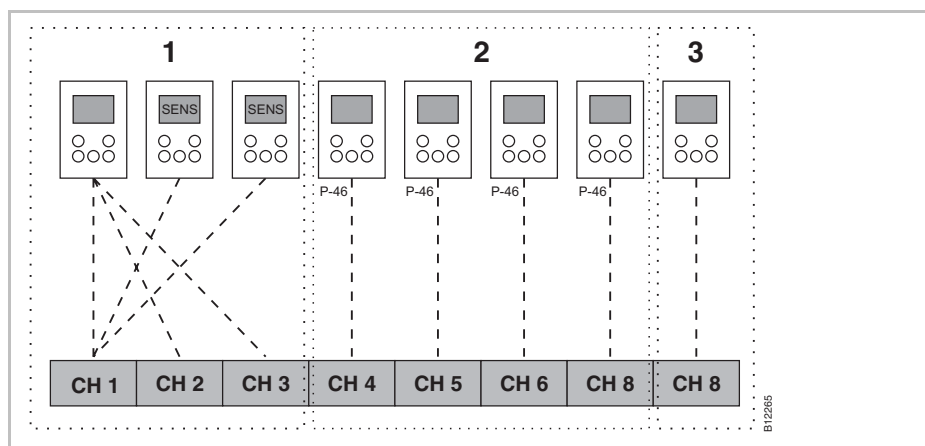
Fig. 47: Radiokanalgrupper med inställning av områden
