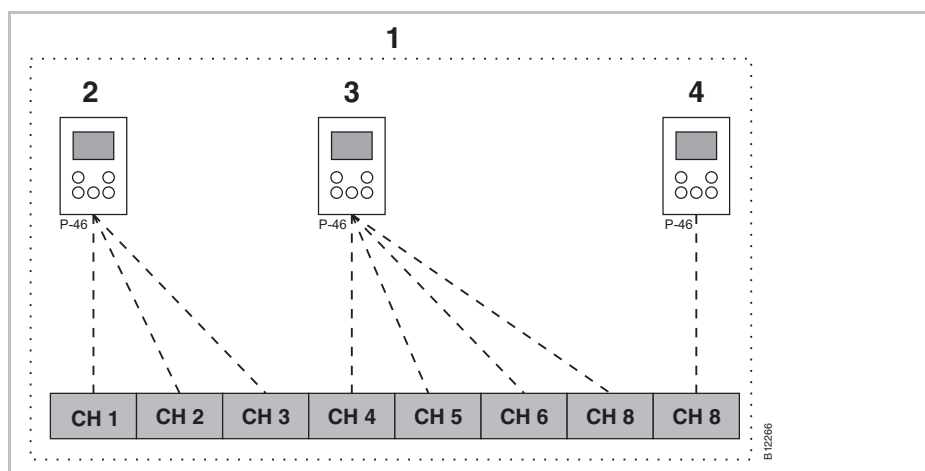
Fig. 48: Delning av inställningspunkt för alla trådlösa rumstermostater i ett område
