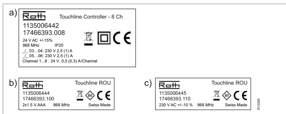
Fig. 1: Märkplåt a) på kontrollenheten, b) på den trådlösa rumstermostaten c) på den trådlösa rumstermostaten, 230 V
