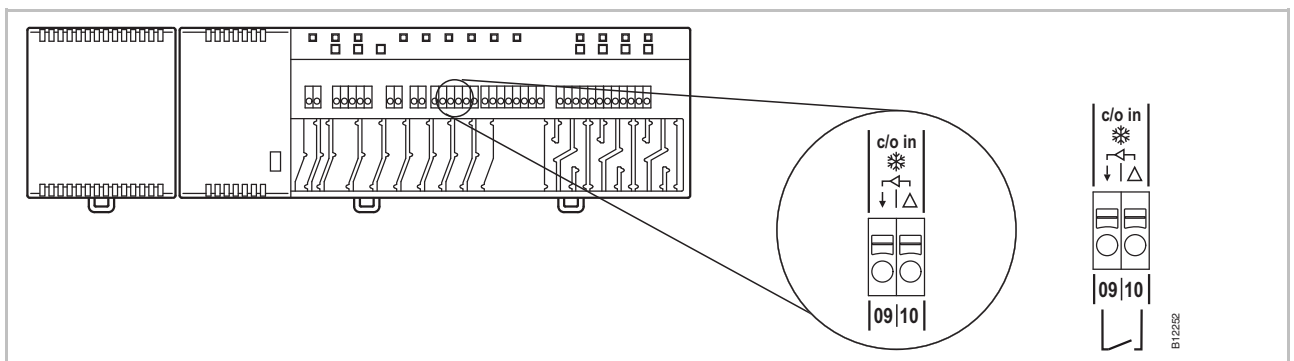
Fig. 29: C/O-ingång, kontaktdetektion
