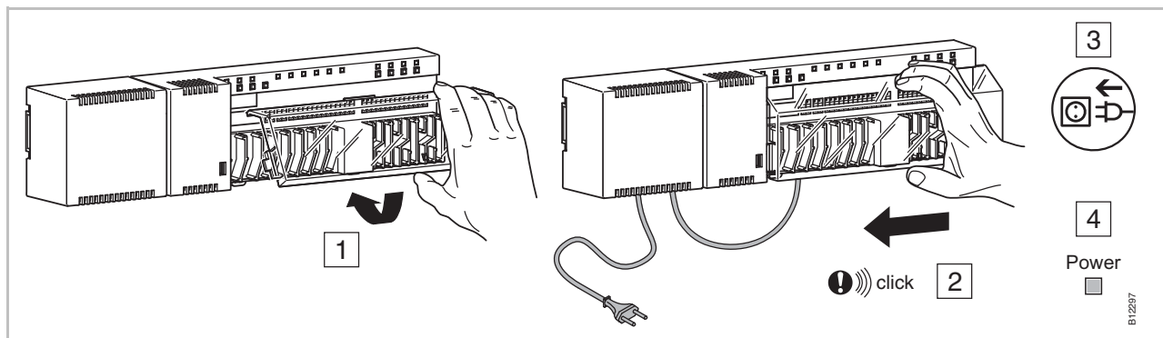
Fig. 33: Montera täckåpan och anslut strömförsörjningen
