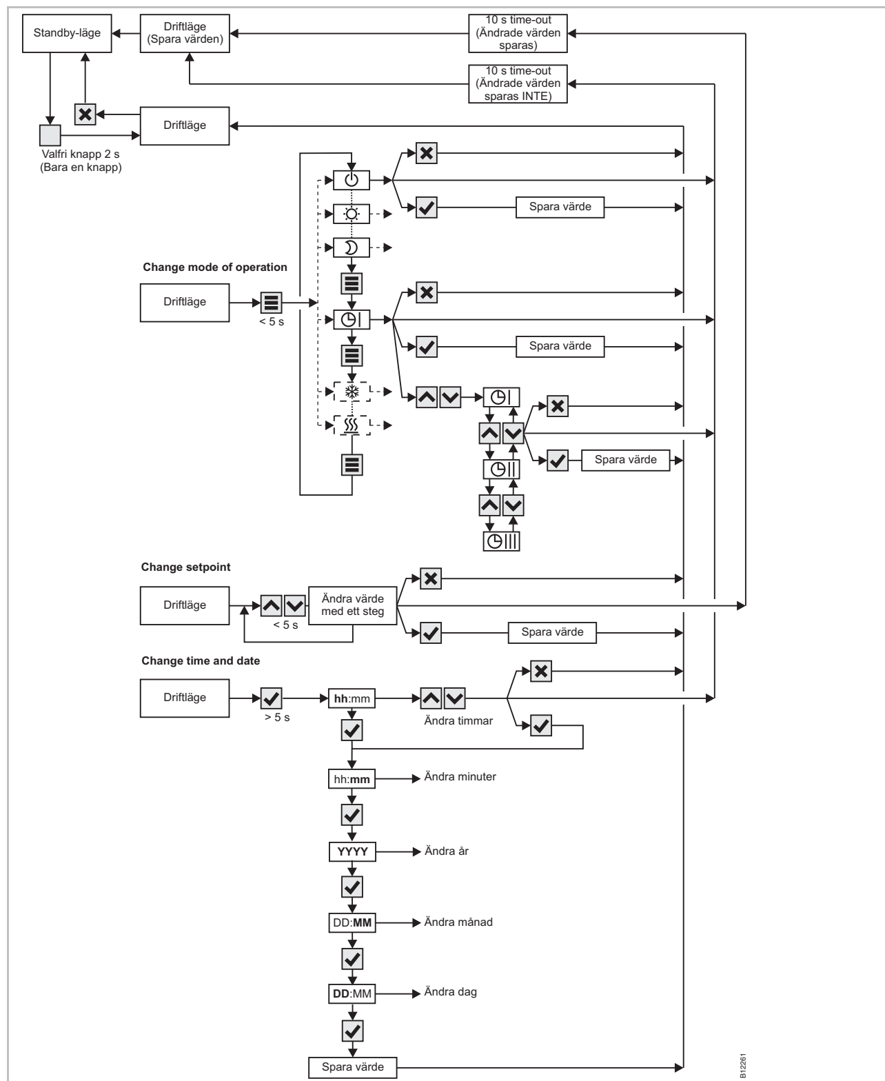
Fig. 43: Menystruktur
