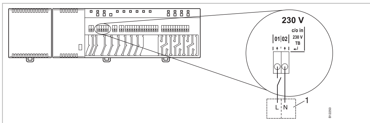
Fig. 27: TB-ingång, kontroll med 230 V
