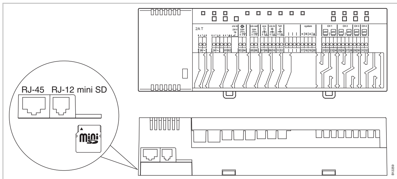
Fig. 38: mini SD-kort
