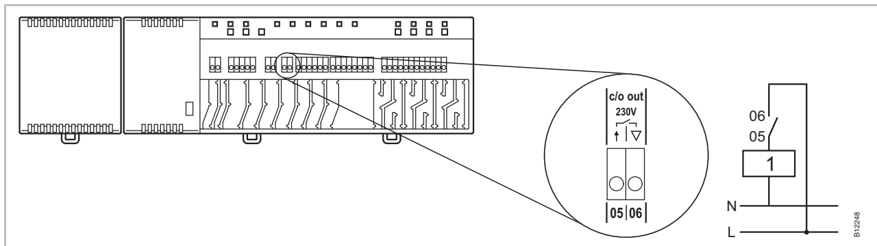
Fig. 24: C/O- eller burner output, 230 V
