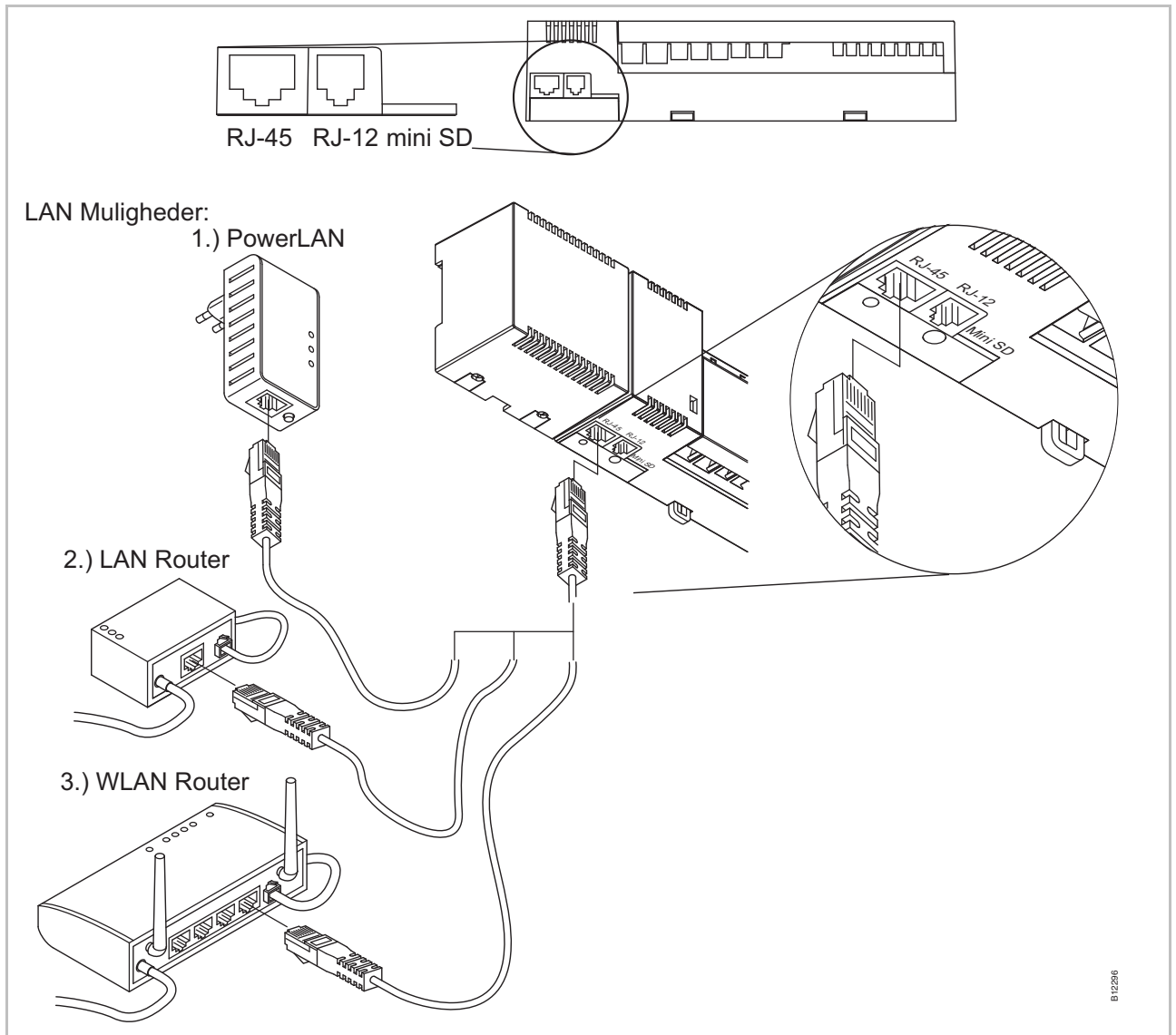
Fig. 32: LAN-nätverk
