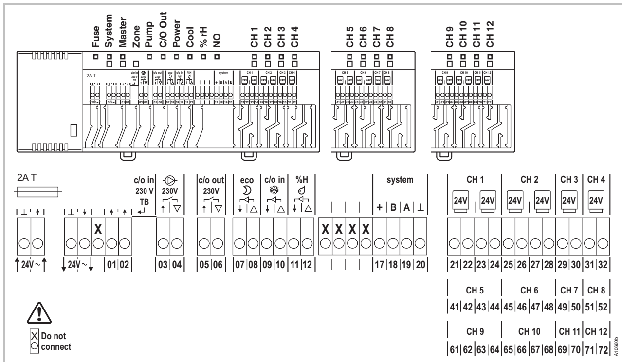
Fig. 19: Kopplingsschema
